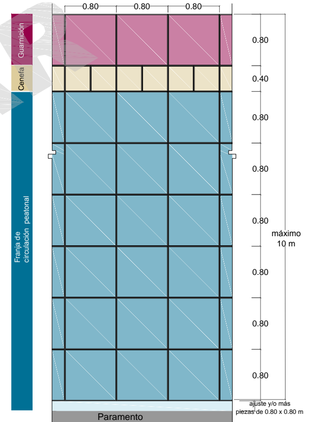
OPCIÓN C - SIN FRANJA DE VEGETACIÓN
