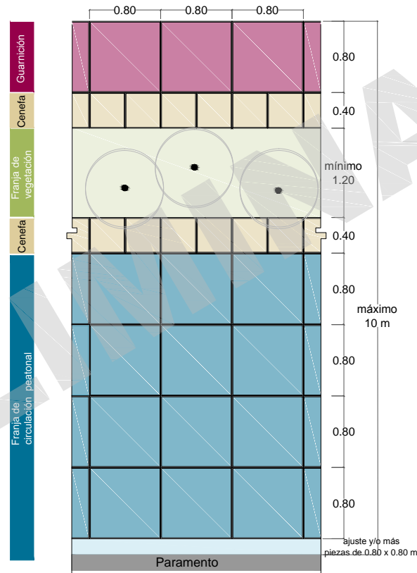
OPCIÓN B- CON FRANJA DE VEGETACIÓN
