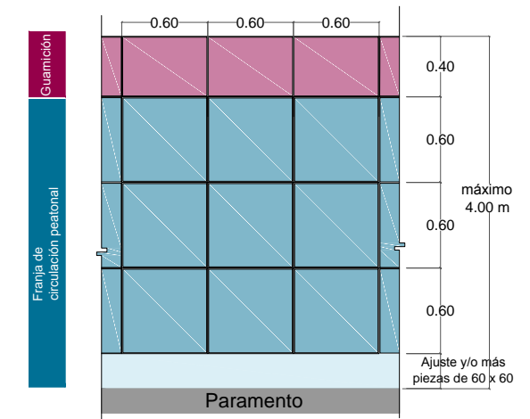
OPCIÓN C - SIN FRANJA DE VEGETACIÓN
