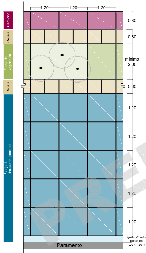
OPCIÓN A - CON FRANJA DE VEGETACIÓN (CAJETES)
