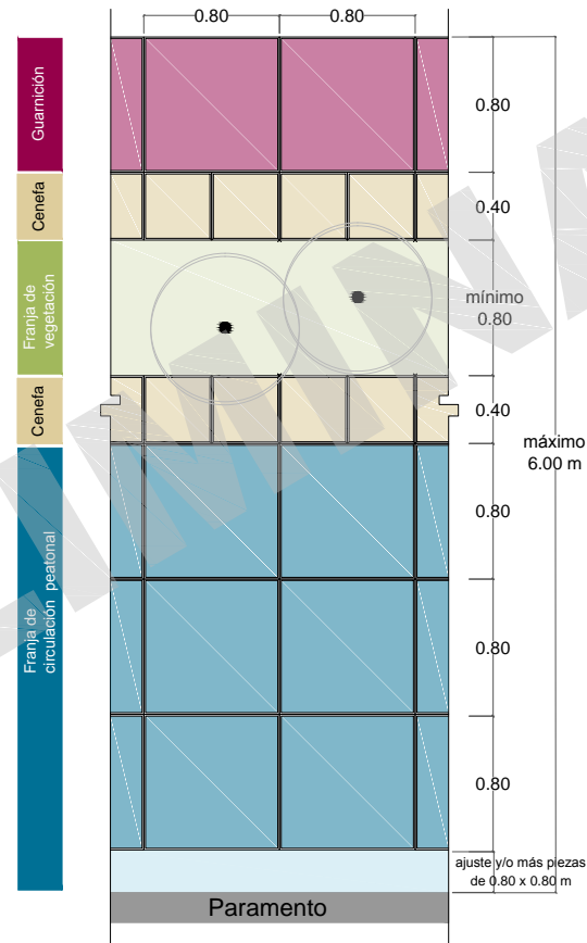
OPCIÓN B - CON FRANJA DE VEGETACIÓN
