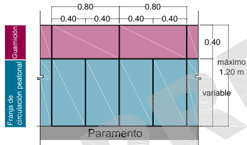
OPCIÓN A - CON GUARNICIÓN 40 CM
