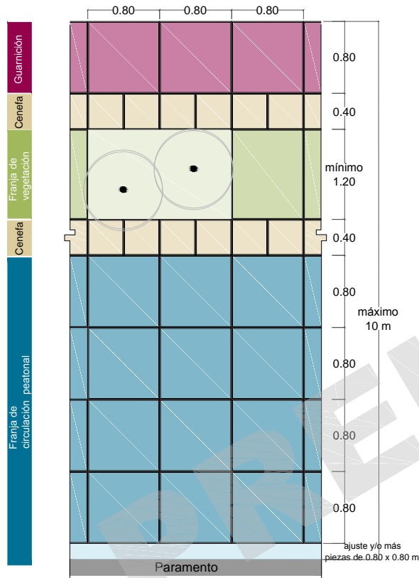
OPCIÓN A - CON FRANJA DE VEGETACIÓN (CAJETES)
