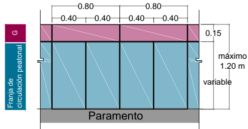
OPCIÓN A - CON GUARNICIÓN 15 CM
